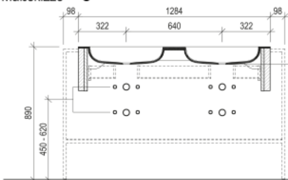
Maßskizze 6
