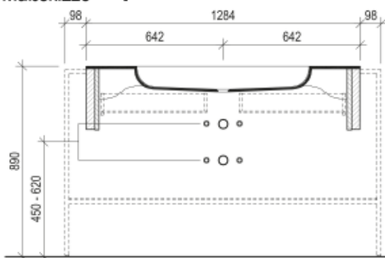
Maßskizze 4
