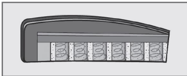
Tonnentaschenfederkern (punktelastischer Tonnentaschenfederkernsitz) abgedeckt mit PUR-Schaum (RG 35).
