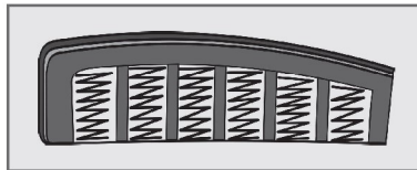
Federkern (gezogener Federstahldraht) abgedeckt mit PUR-Schaum (RG 35).
