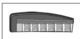
Tonnentaschenfederkern (punktelastischer Tonnent- taschenfederkernsitz) abgedeckt mit PUR-Schaum (RG 35).
